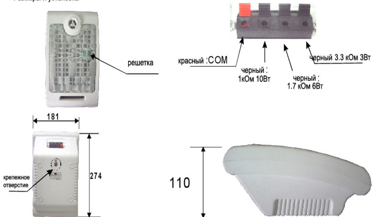
Размеры и установка
