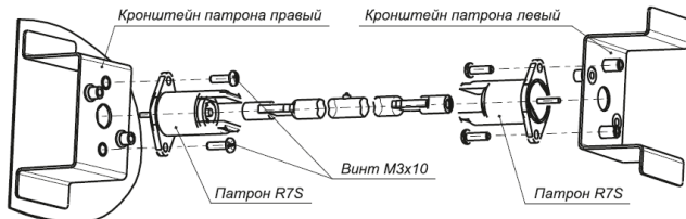
Рисунок 7 Установка патронов под лампу длиной 132мм
