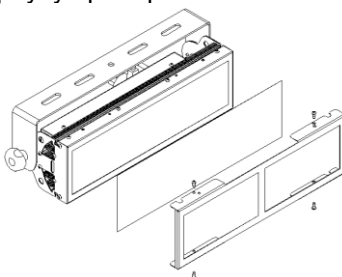
Рисунок 4 Схема установки светофильтра
