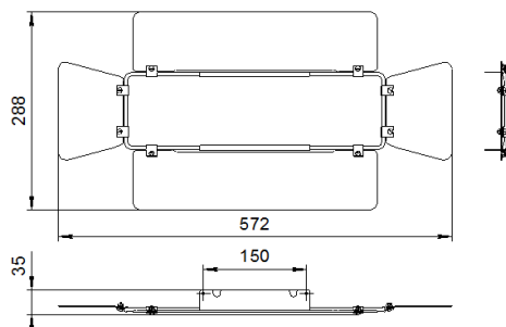
Рисунок 2 Габаритный чертеж Шторки кашетирующие FL LED 60
