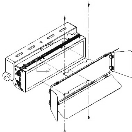
Рисунок 3 Схема установки шторок кашетирующих
